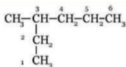
3 - ميثيل هكسان
