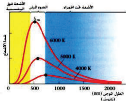
يتناسب الطول الموجي لقمم المنحني عكسيا مع درجة الحرارة
