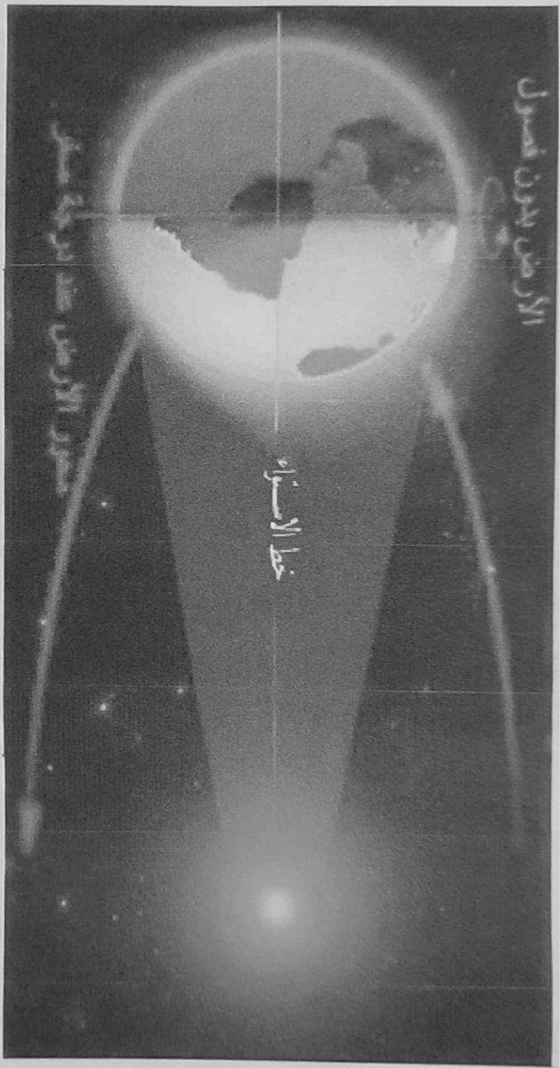
الشكل (١٧) محور الأرض افترضاً عمودي
