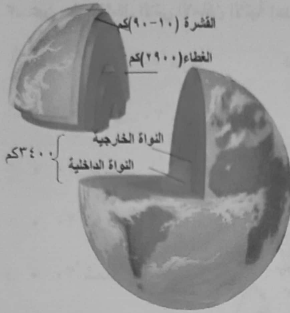
الشكل (١١) بنية الأرض
